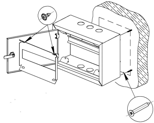
Рис.1. Схема монтажа
