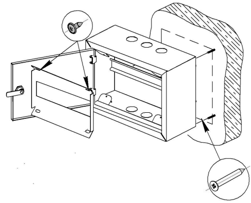
Рис.1. Схема монтажа
