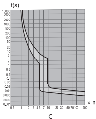
Время-токовые характеристики УЗДП
