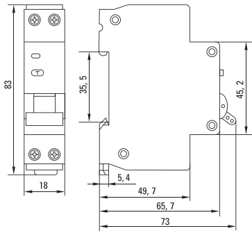
Рис. 2 Габаритные размеры АВДТ-63М
