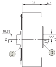
3 Разделительная пластина
