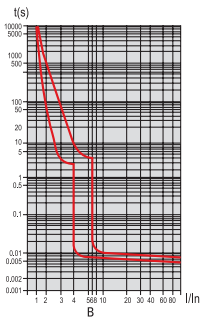
Рис. 1. Время-токовые характеристики
