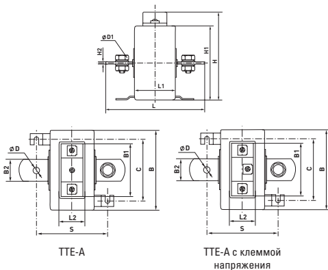
Рисунок 1 – Габаритные и установочные размеры модификаций ТТЕ-А
