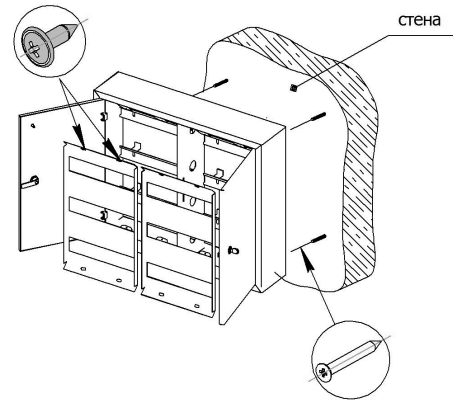
Рис.1. Схема монтажа
