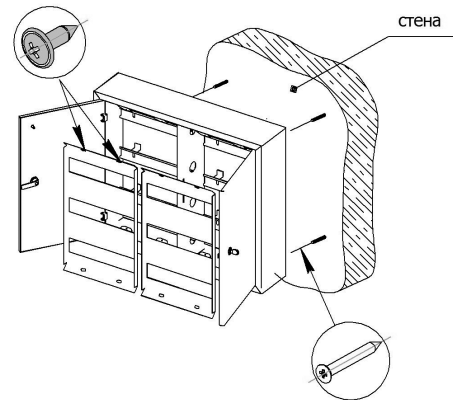
Рис.1. Схема монтажа
