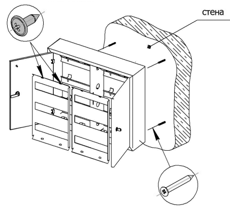
Рис.1. Схема монтажа
