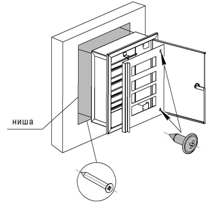
Рис.1. Схема монтажа
