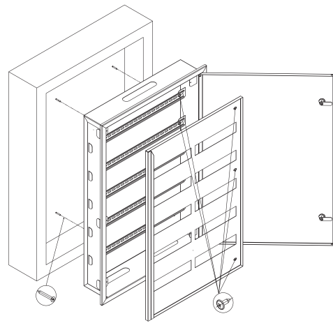
Рис.1. Схема монтажа
