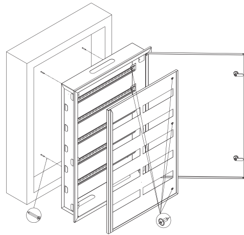
Рис.1. Схема монтажа
