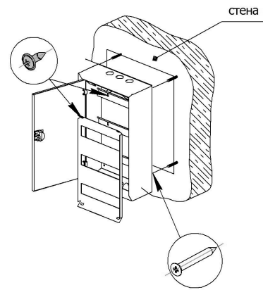
Рис.1. Схема монтажа
