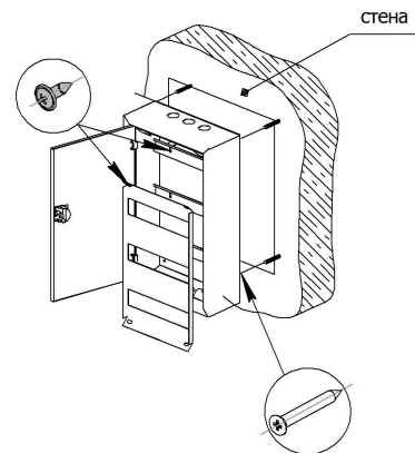
Рис.1. Схема монтажа
